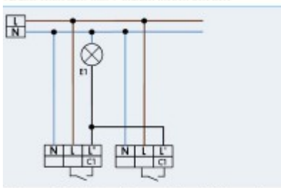
Schema zapojení detektoru pohybu pro paralelní spojení více senzorů pohybu. Maximální počet paralelně zapojených senzorů je třeba vždy prověřit předem.
