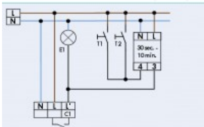
Schema zapojení detektoru pohybu ve spojení s tlačítkovým časovým automatem například ve schodišťových aplikacích.
