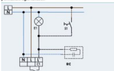
Schema zapojení detektoru pohybu pro funkci trvalého zapnutí tlačítkem. Funkce se zapne/vypne stiskem tlačítka S1.
