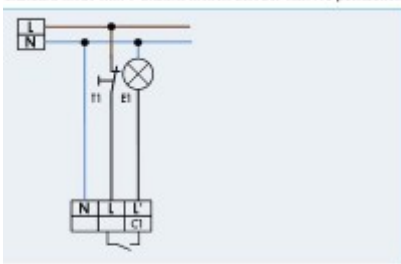
Schema zapojení pro ruční reset tlačítkem pohybu. Funkce se posílá v případě, kdy došlo například k nedokonalému výpadku sítě 230V a po obnovení napájení čidlo zůstalo po vypršení nastaveného času sepnuto. Reset se spustí stiskem tlačítka T1 na dobu cca 2sec.
