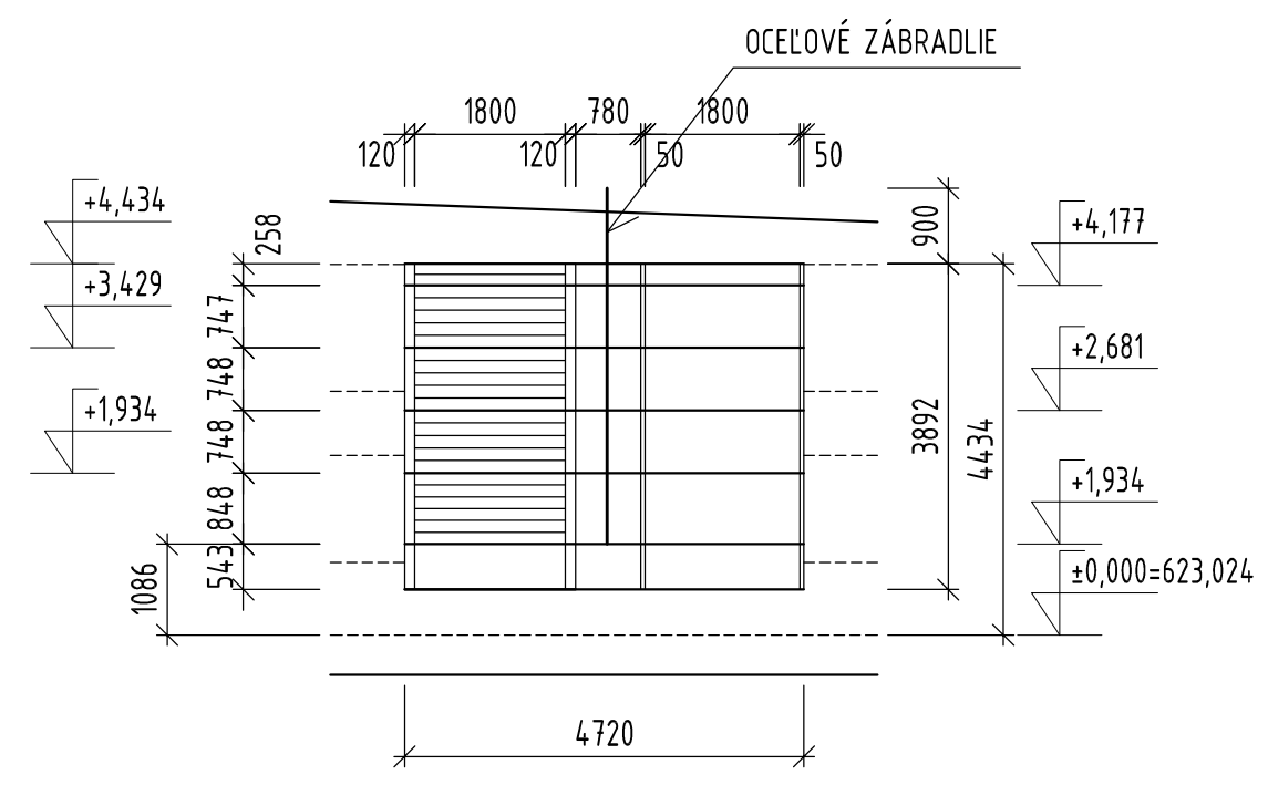
POHLAD ZÁPADNÝ M=1:100
